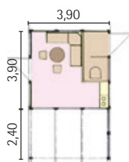
Größe 1, 15 m 2 Vordach
