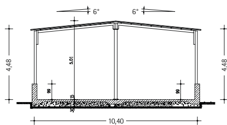
Querschnitt
