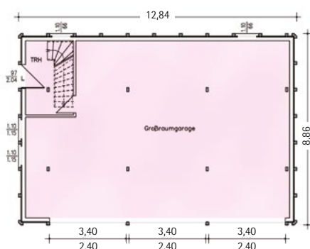
Erdgeschoss Großraumgarage/Werkstatt, 100 m² Nutzfläche mit drei großen Sektionaltoren und innenliegendem Treppenhaus
